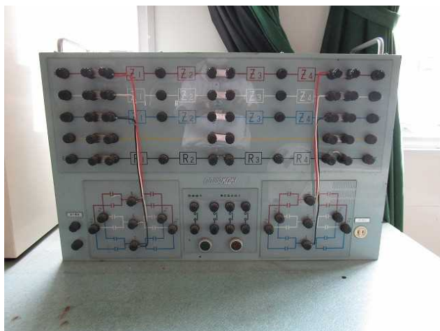
①模擬送電線実習装置 1 台
